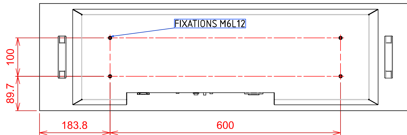
VUE ARRIERE
