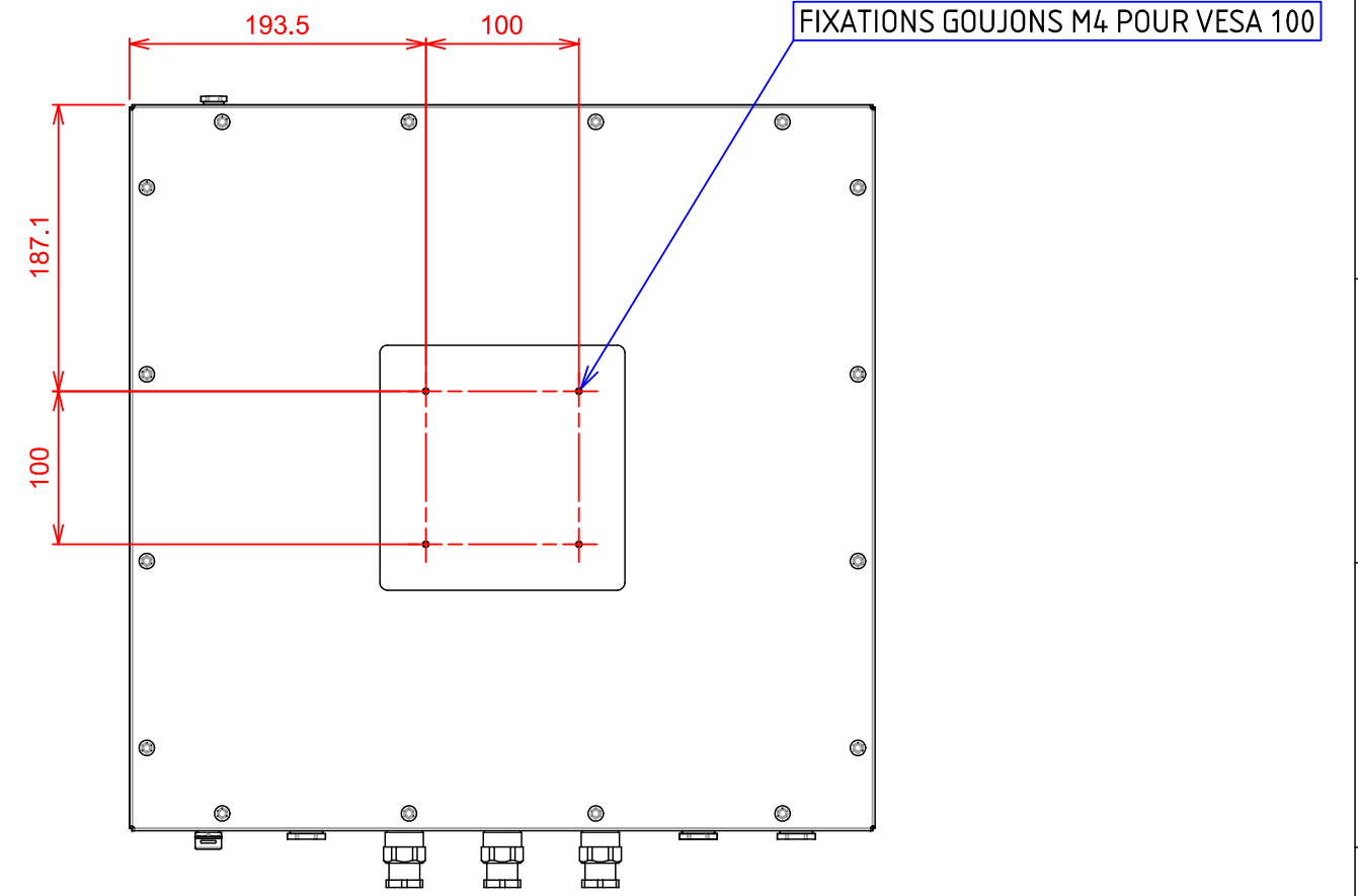
VUE ARRIERE
